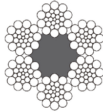
6x26 ws AF
