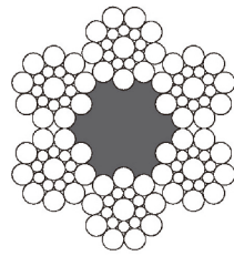
6x19 s AF
