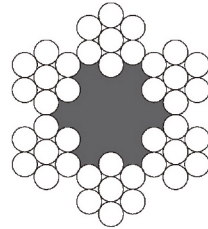
6x7 AF
